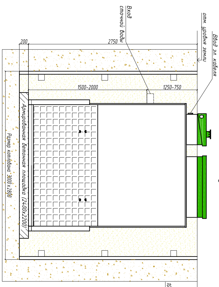
Вид сбоку
